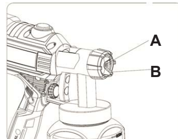
Чищення сопла А та повітряного ковпачка В
