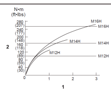
Правильний момент затягування для високоміцного болта.
