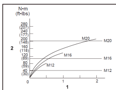
Правильний момент затягування для стандартного болта.
