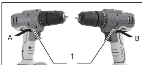
1. Кнопка перемикачання реверса
